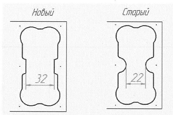
Рисунок 1. Доработка посадочного отверстия
