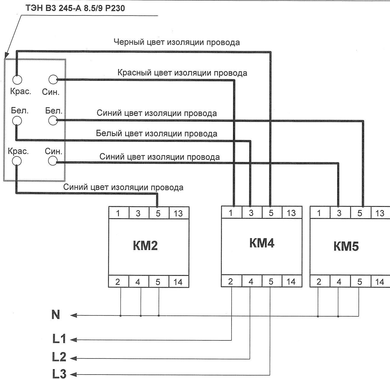
Рисунок 2. Схема подключения ТЭНа В3 245-А 8.5/9 Р230
