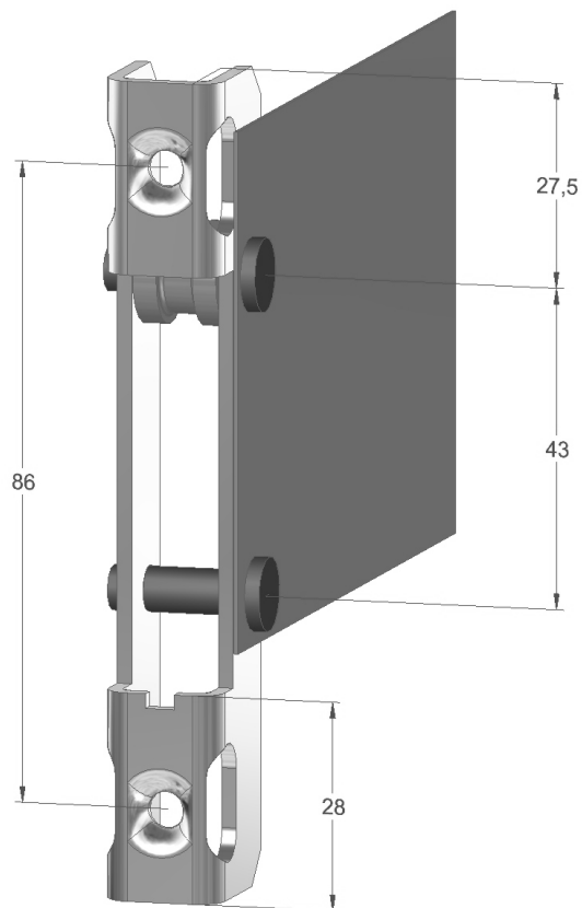
Контрпетля для запасных частей
