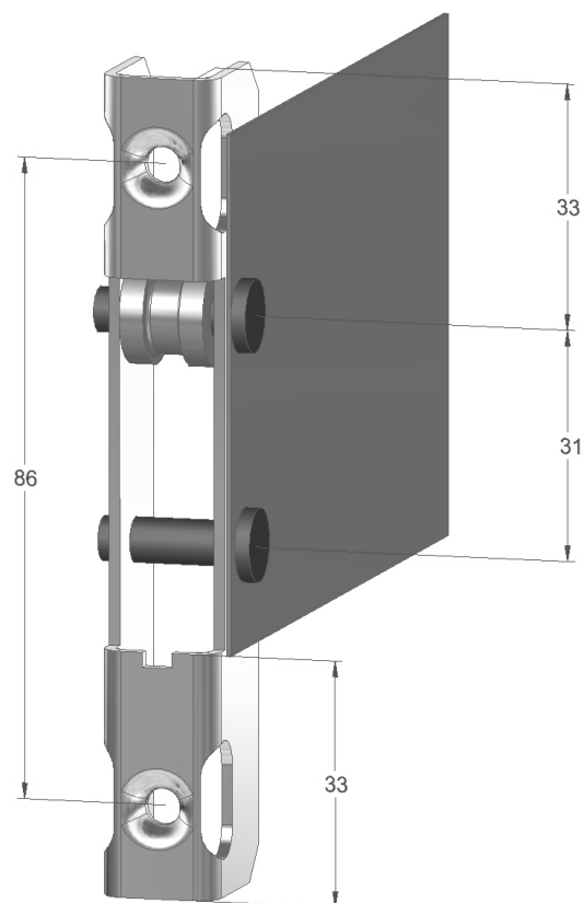
Контрпетля для серийных изделий
